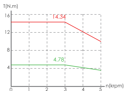
MV7E-M11A-1R530-□□
