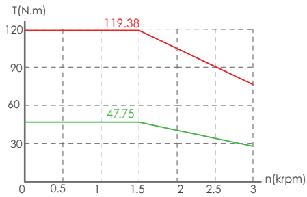
MV7E-M18-7R515-□□H
