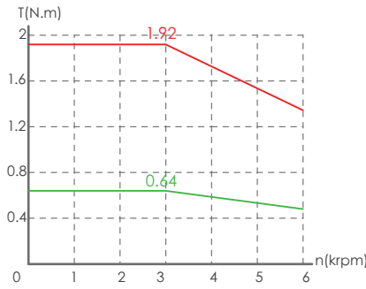
MV7E-L06A-R2030-□□
