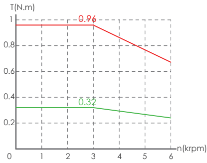
MV7E-L04A-R1030-□□
