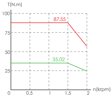
MV7E-M18-5R515-□□
