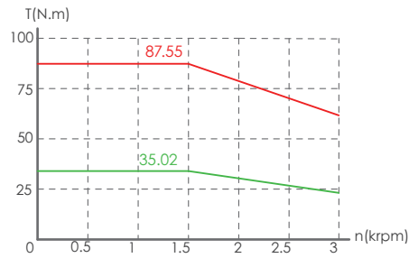
MV7E-M18-5R515-□□H
