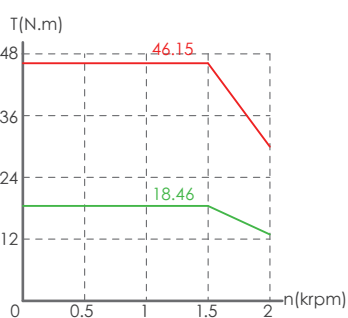
MV7E-M18□-2R915-□□
