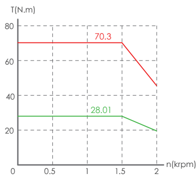
MV7E-M18□-4R415-□□
