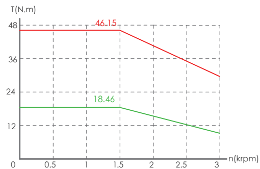
MV7E-M18□-2R915-□□H
