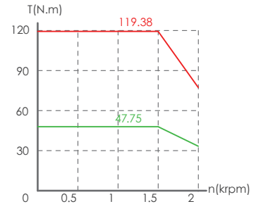
MV7E-M18-7R515-□□
