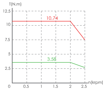
MV7E-L08A-R7520-□□ L
