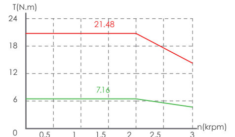
MV7E-M13-□1R520-□□
