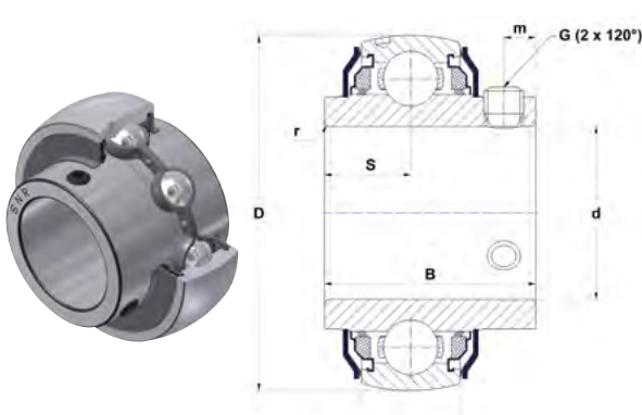
UC2..AGR
