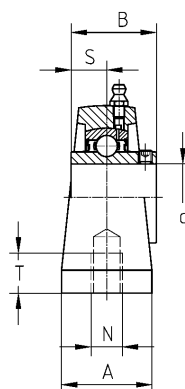
SUCPA200
