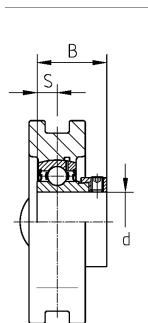
SEST200
