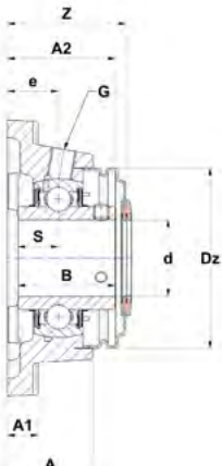
UCFE..CO
