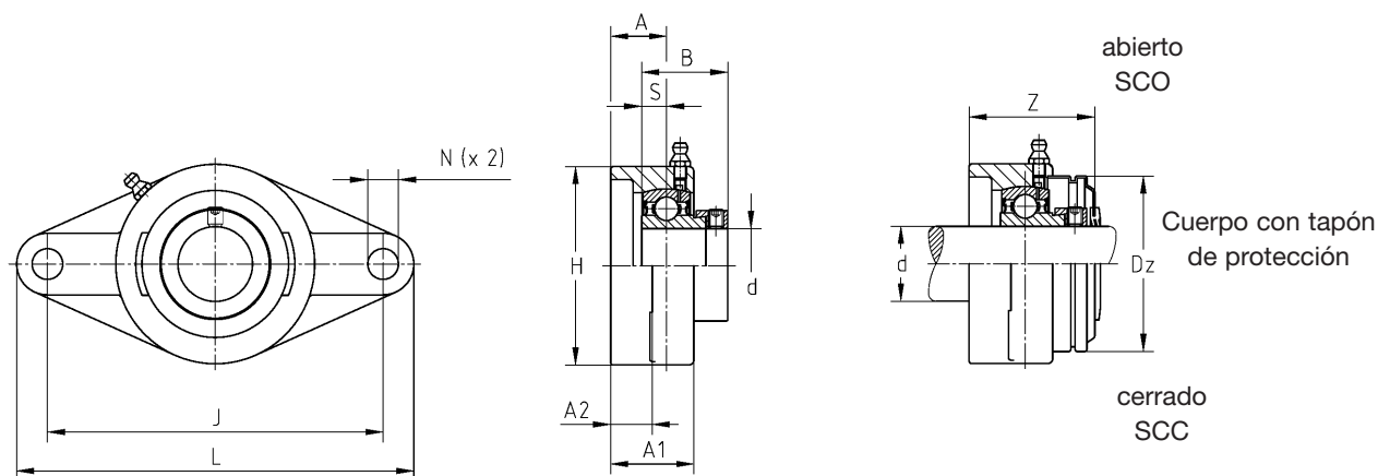
SESFL200
