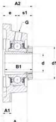
UKFE..H
