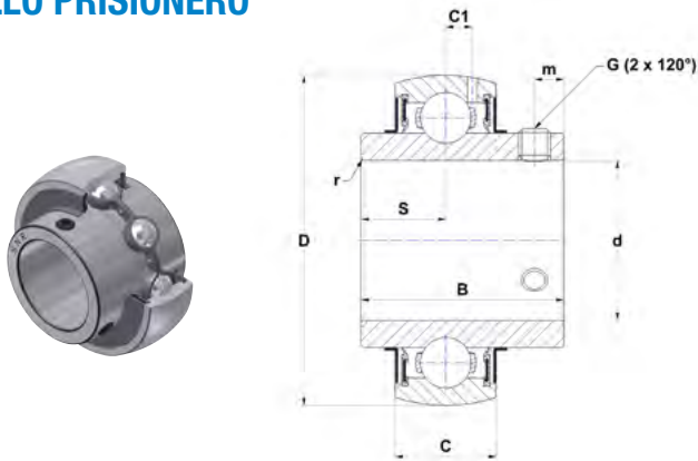
UC..G2
