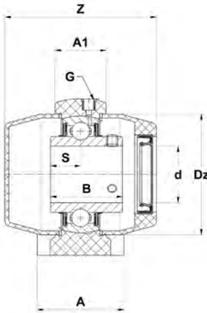
MUCPPL + Tapas protectoras
