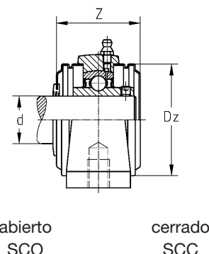
Cuerpo con tapón de protección
