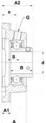
USFE
