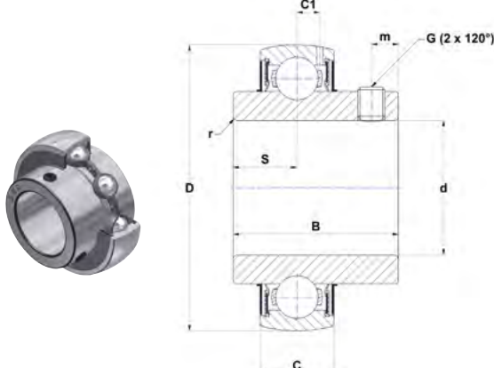
UCX..G2
