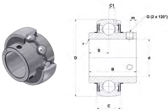
UC..G2
