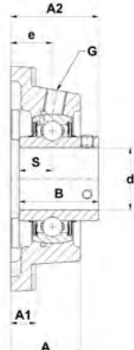
UCFE
