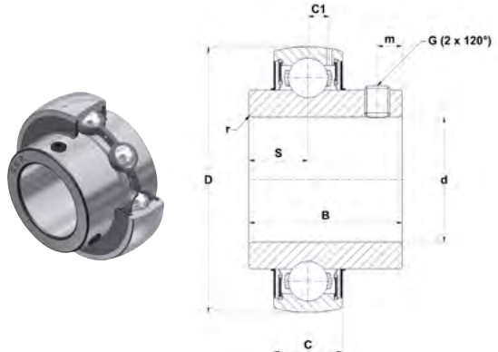
UCX..G2
