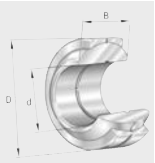
GE...-HO-2RS
